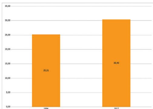
Évolution de l'indice de méditerranéité moyen du cortège des passereaux nicheurs de la réserve naturelle du Mas Larrieu
