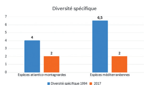
Évolution de la diversité spécifique des espèces très méditerranéennes (IM fort) et des espèces peu méditerranéennes (IM faible) entre 1994 et 2017.
