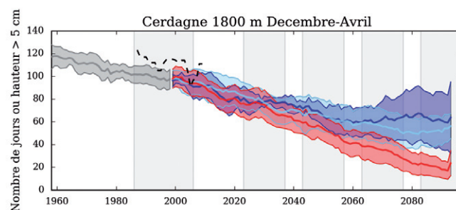
Figure 2 : Évolution du nombre de jour de neige au sol en Cerdagne (altitude 1800m) selon les projections Eurocordex (source projet Clim'Py) : scénario historique en gris, observations en noir pointillé, scénario d'émissions fortes en rouge, d'émissions modérées en bleu clair, d'émissions faibles en bleu foncé.
