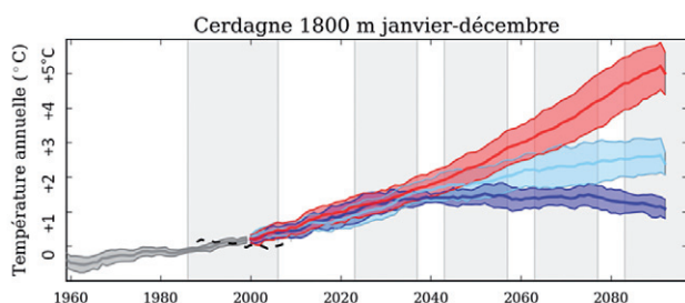
Figure 1 : Évolution des températures moyennes annuelles en Cerdagne (altitude 1800m) selon les projections Eurocordex (source projet Clim'Py) : scénario historique en gris, observations (1986-2005) en noir pointillé, scénario d'émissions fortes en rouge, d'émissions modérées en bleu clair, d'émissions faibles en bleu foncé.
